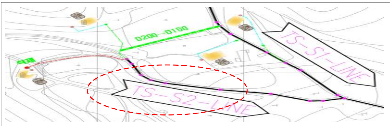
[그림 3] 송골지역 S2라인 배수설비 계획
