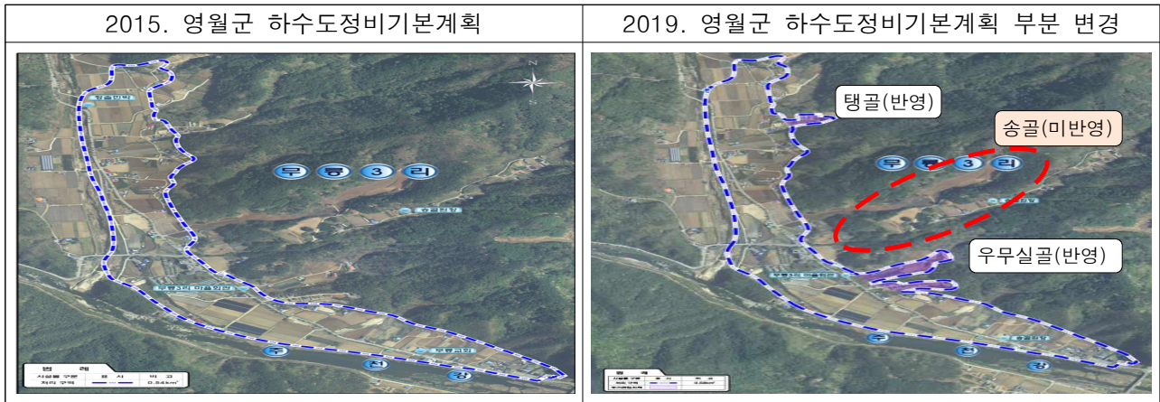
[그림 1] 영월군 하수도정비기본계획 부분변경 처리구역도
