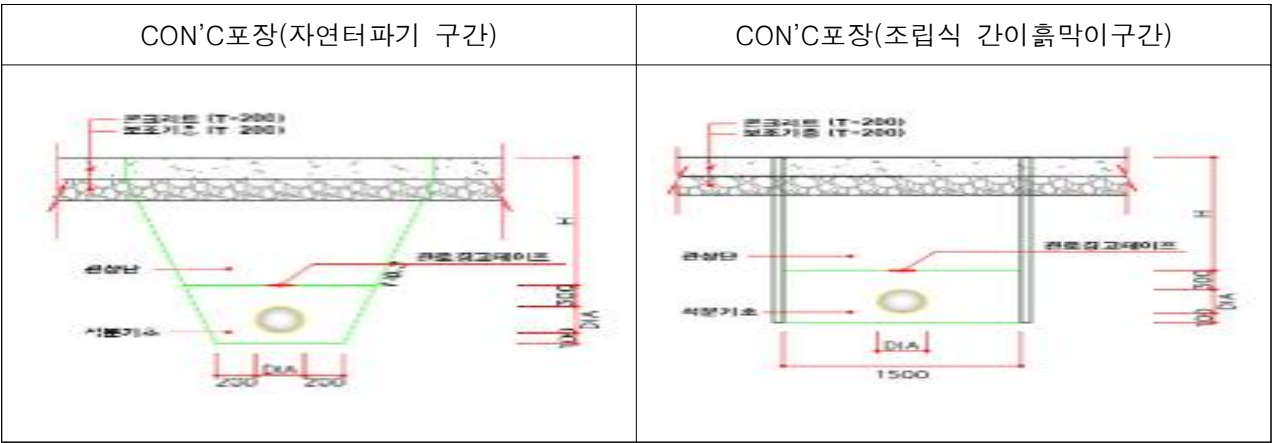
[그림 2] 송골구간 포장복구 계획 단면도
