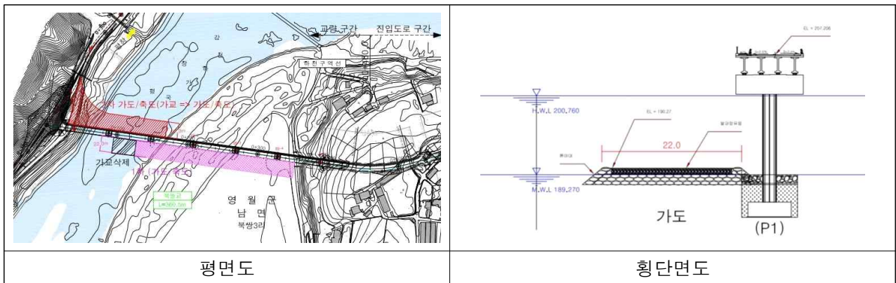
[표 3] 공사용 가도 대체방안
