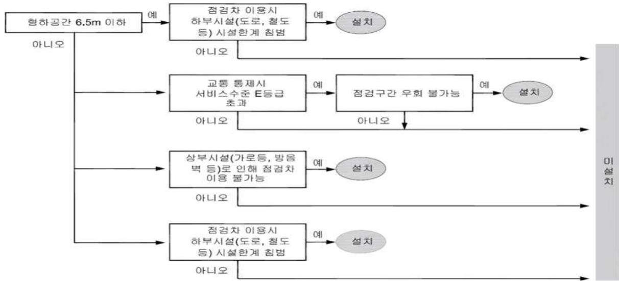
[그림1] 교량 점검통로 설치 의사결정 흐름도(2차로 초과)
